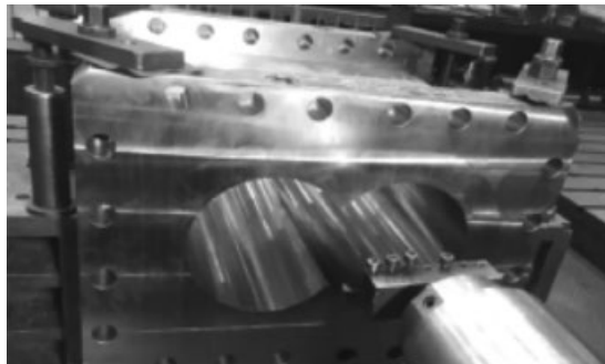
图 4 数控镗床加工
