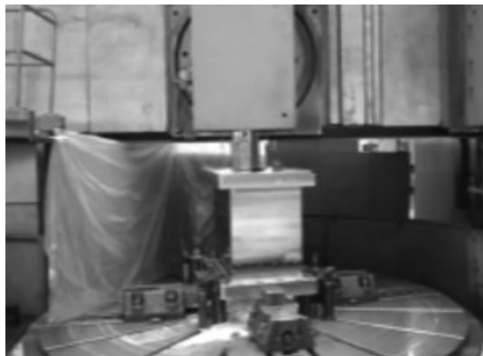
图 3 数控立车磨削机筒内孔
