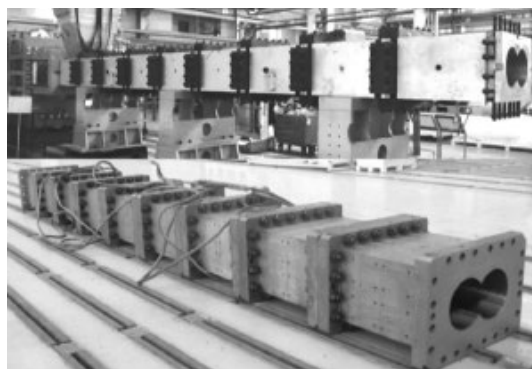
图1 同向造粒机组机筒串联组装图
